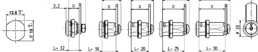
DIMENSIONI FORO DI FISSAGGIO CUT-OUT - EINBAUÖFFNUNG - PERÇAGE
