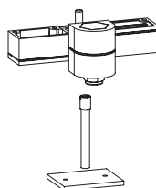
Cerniera UNITAS 93 Bo con perno e piastra d'appoggio 6-25851-00-P-*
