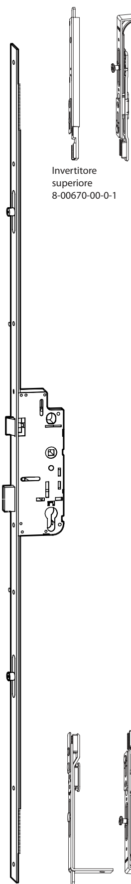
Giunto inferiore con uscita chiusura 8-00676-00-0-1
