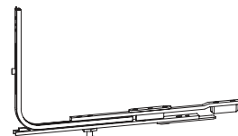
Chiusura K 160.2 Se 6-28604-00-0-1 nottolini in acciaio
