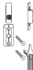
Maniglia estraibile E-18333-00-0-7 Rosetta con copertura G-46231-00-0-7 Scontro E-13880-00-0-7 Vite TS M 5 x 35 9-13255-35-0-1
