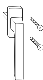
Maniglia DIRIGENT-F 6-28072-29-0-7 Vite TS M 5 x 40 9-13255-40-0-1
