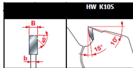
HW K10S Tooth features - Caratteristiche del dente
